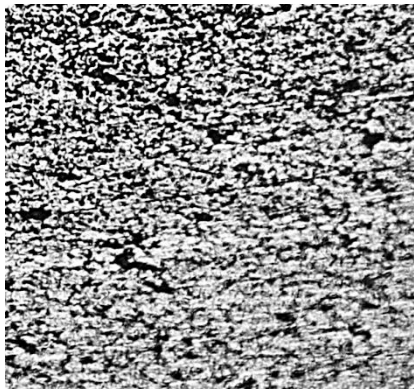
Рис. 3. Мікροструктура сплаву АМг6 за \omega = 1\ 250\ \text{хв}^{-1} залежно від температури перемішування, збільшення 500: a – 330 °C; б – 345 °C; в – 360 °C
