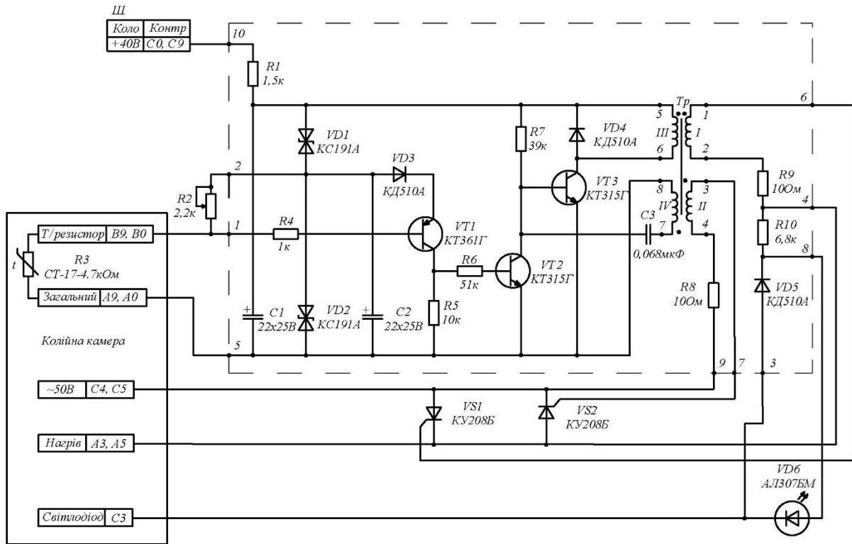
Рис. 1. Принципова схема терморегулятора ТРМ
