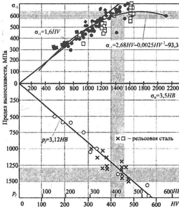
Рис. 1. К анализу взаимосвязей характеристик сопротивления усталости, твердости и предела прочности
