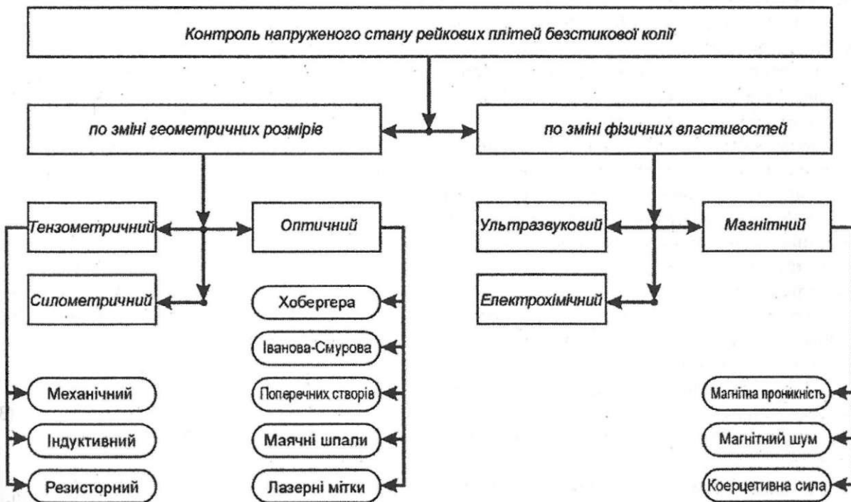
Рис. 1. Класифікація методів контролю напружень в рейкових плітях
