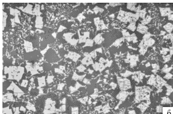
Рис. 5. Мікроструктура вкладиша підшипника з бабіту Б16, отриманого відцентровим литтям (зона 2); світлі включення – зміцнюючі фази SnSb і \text{Cu}_3\text{Sn} , окремі голки – \text{Cu}_2\text{Sb} ; темні ділянки – твердий розчин на основі свинцю, x125: а – \approx 4600 \text{ мкм} ; б – \approx 5200 \text{ мкм} (від краю контактної взаємодії)
