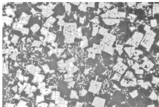
Рис. 4. Мікроструктура вкладиша підшипника з бабіту Б16 біля краю контактної взаємодії отриманого відцентровим литтям (зона 1), x125
