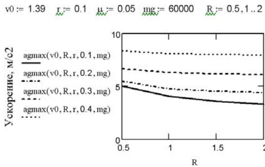
Рис. 3. Зависимость максимального ускорения груза от радиуса опорных поверхностей R (катковые ТКУ)
