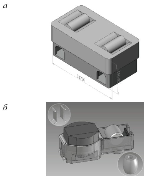
Рис. 6. Варианты исполнения боковых скользунов постоянного контакта: а) типа подрессоренный ролик; б) упруго-роликовый скользящий ФГУП «ПО «Уралвагонзавод» с антифрикционной накладкой на контактной поверхности
