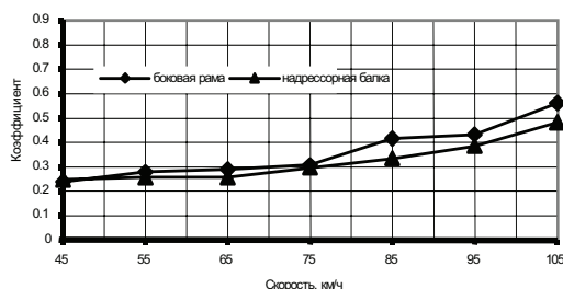
Рис. 4. Максимальный (с вероятностью 99,9 %) коэффициент вертикальной динамики, измеренный по боковой раме и наддрессорной балке на прямом участке пути для вагона на тележках-прототипах
