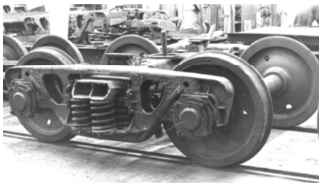
Рис. 1. Общий вид тележек УВЗ-ЛИИЖТ (а), УВЗ-6КМ (б) и 50X-508 (в), в создании и испытаниях которых принимали участие В. А. Лазарян и И. И. Челноков
