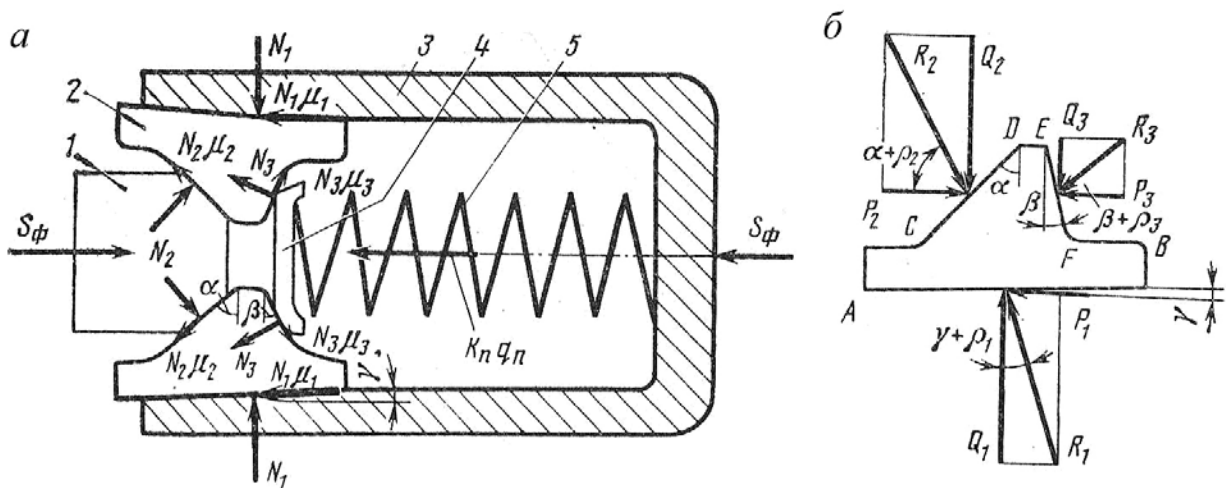
Рис. 3. Розрахункова схема поглинального пружинно-фрикційного апарату (а) та сили, що діють на клин (б)
